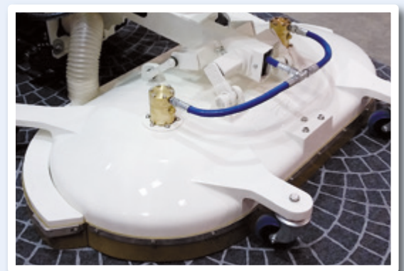
Elastische Lagerung für Strassenwischmaschine.
