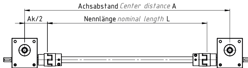
Korrekturmaß Achsabstand Ak correction dimension center distance Ak [mm]
