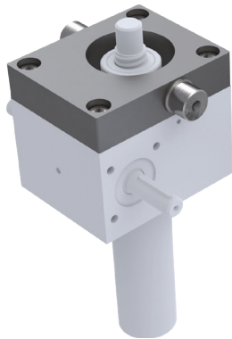
Anbauseite F Attachment side F
