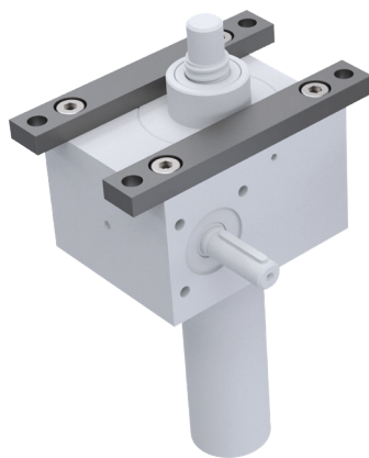
Anbauseite F Attachment side F
