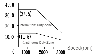
Torque(Nm)
