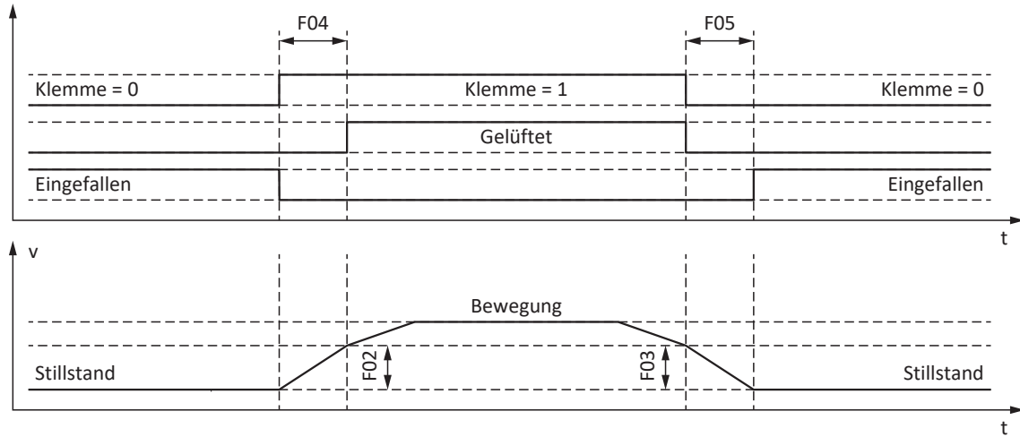
Abb. 52: Bremsenansteuerung bei Steuerart B20 = 0: ASM - U/f-Steuerung oder 1: ASM - U/f-Schlupfkompensiert
