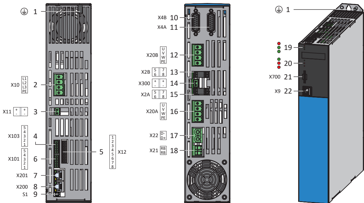
Abb. 28: Anschlussübersicht am Beispiel SC6A162
