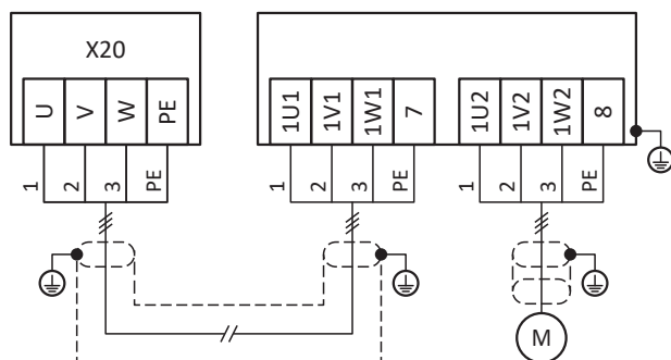
Abb. 54: Anschlussbeispiel Ausgangsdrossel TEP
