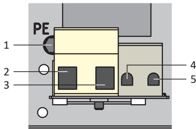
Abb. 52: Anschlussübersicht FZZMQU
