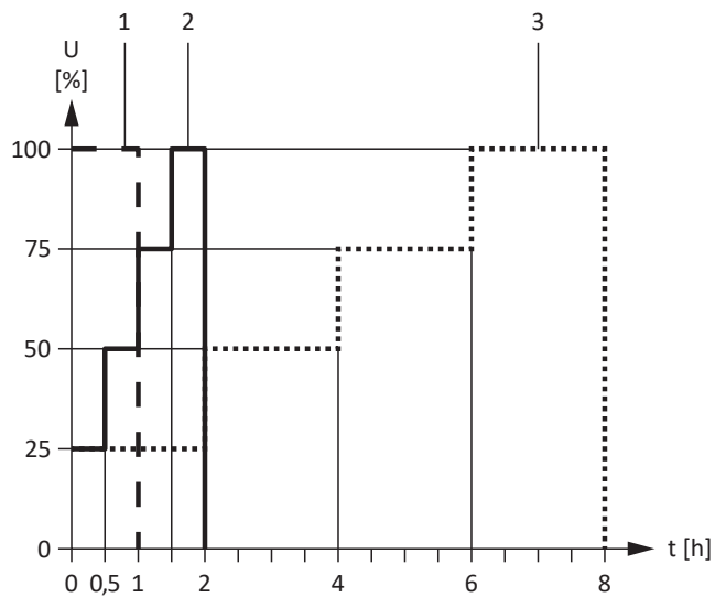
Abb. 31: Spannungshöhen in Abhängigkeit von der Lagerungszeit
