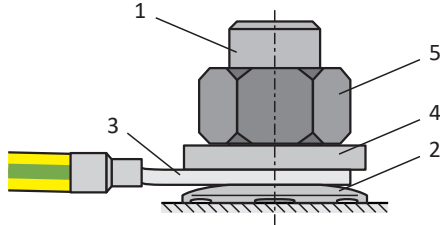
Abb. 44: Anschluss des Schutzleiters
