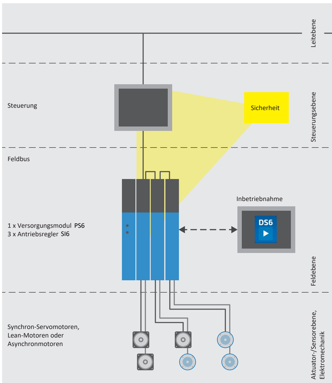
Abb. 2: Systemüberblick zur Anreihtechnik mit SI6 und PS6
